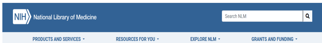
Slika 1: NLM pretraživač
